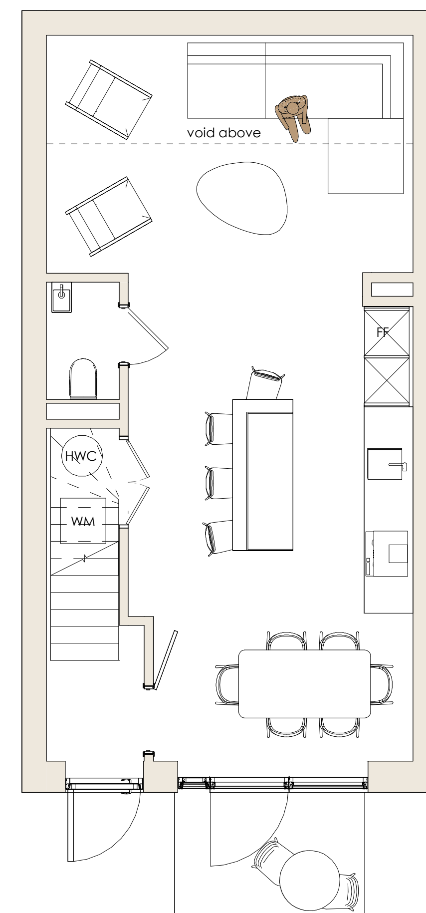
PLANS: G 1:50
